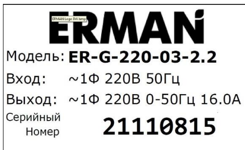
Пример шильдика
