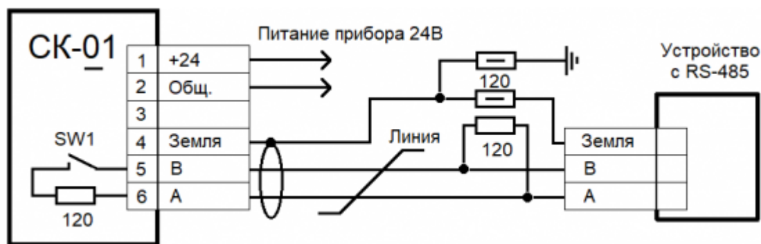
Рисунок 4 - Схема подключения линии RS-485 (с дренажным проводом)
