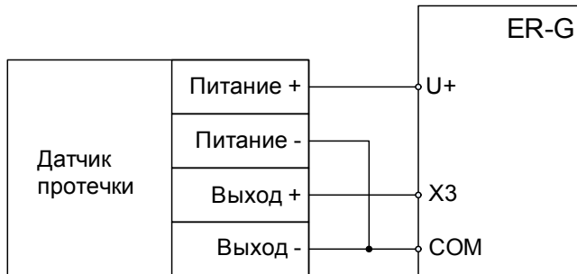
Рисунок 10 – Подключение внешнего датчика протечки
