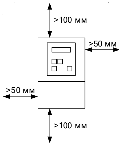
Рисунок 3 – Установка ПЧ
